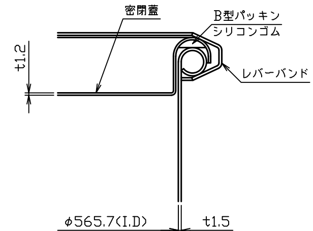
A部詳細図 S = 1 : 2
