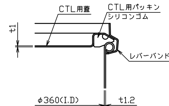
A部詳細図 S = 1 : 2
