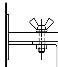
蝶ボルト部詳細図 S = 1 : 2
