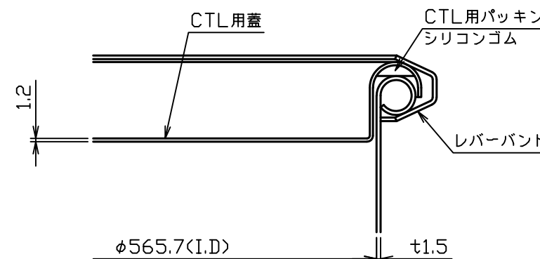
A部詳細図 S = 1 : 2
