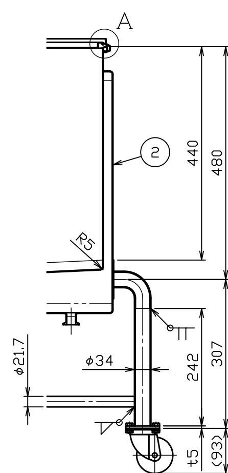
A部詳細図 S = 1 : 1
