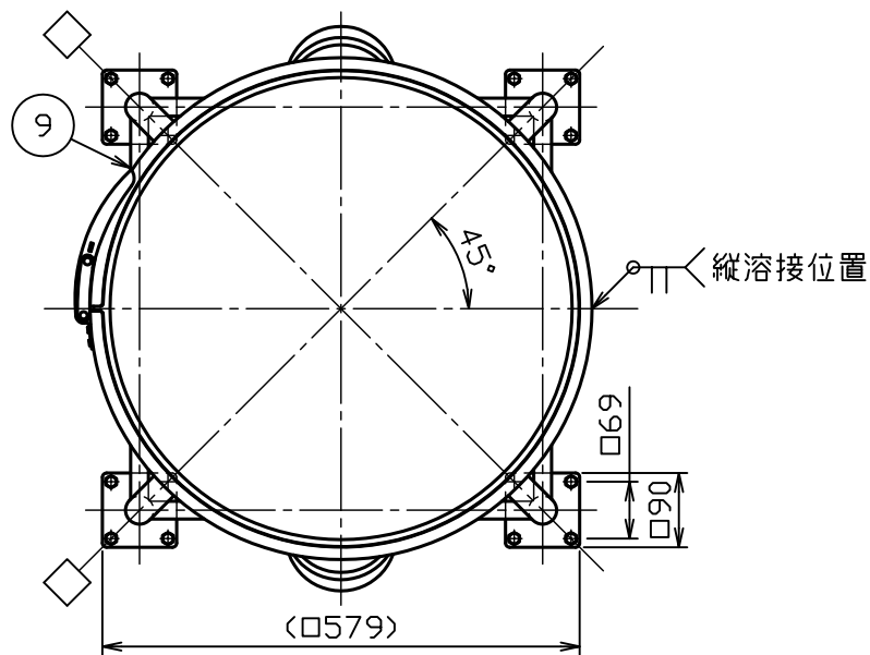
A部詳細図 S = 1 : 1
