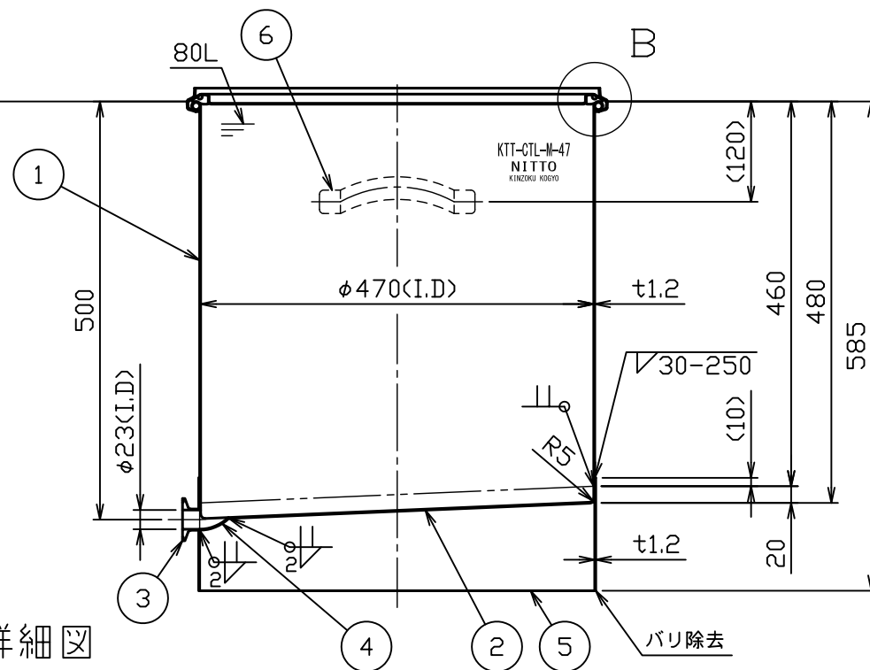
A-A断面図
