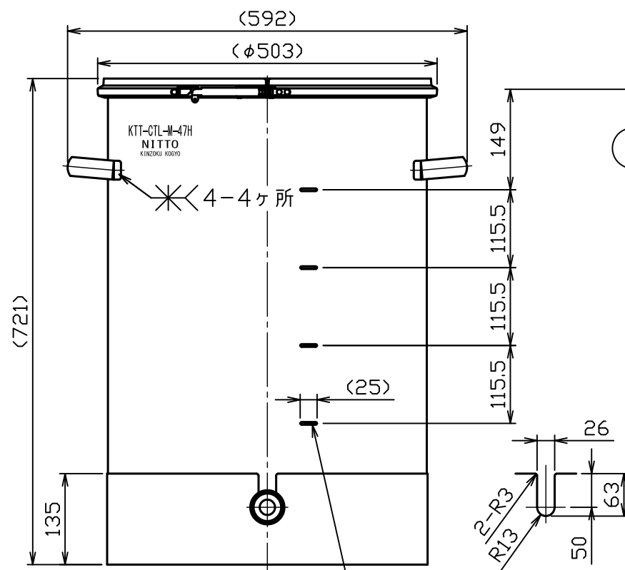
袴切り欠き詳細図
