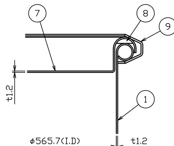
B部詳細図 S = 1 : 2
