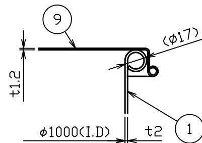
A部詳細図 S = 1 : 3
