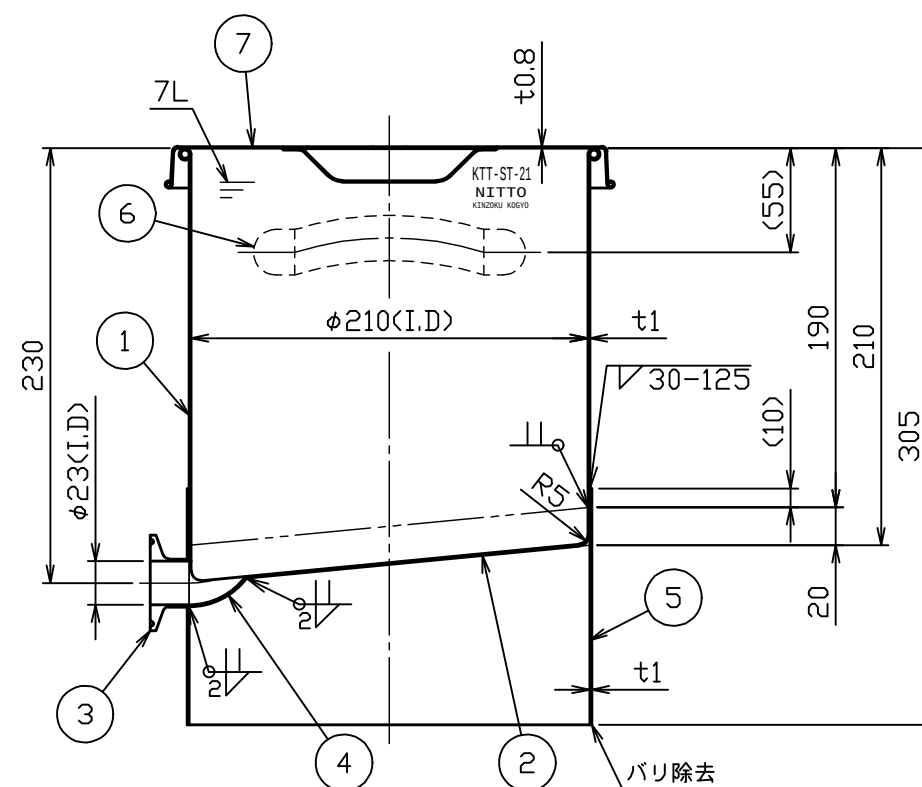
A-A断面図
