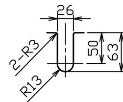
袴切り欠き詳細図
