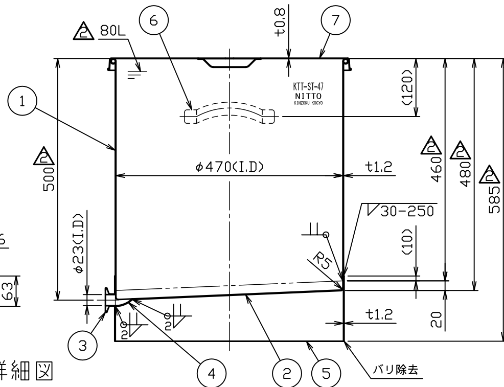
A-A 断面図
