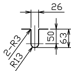
袴切り欠き詳細図
