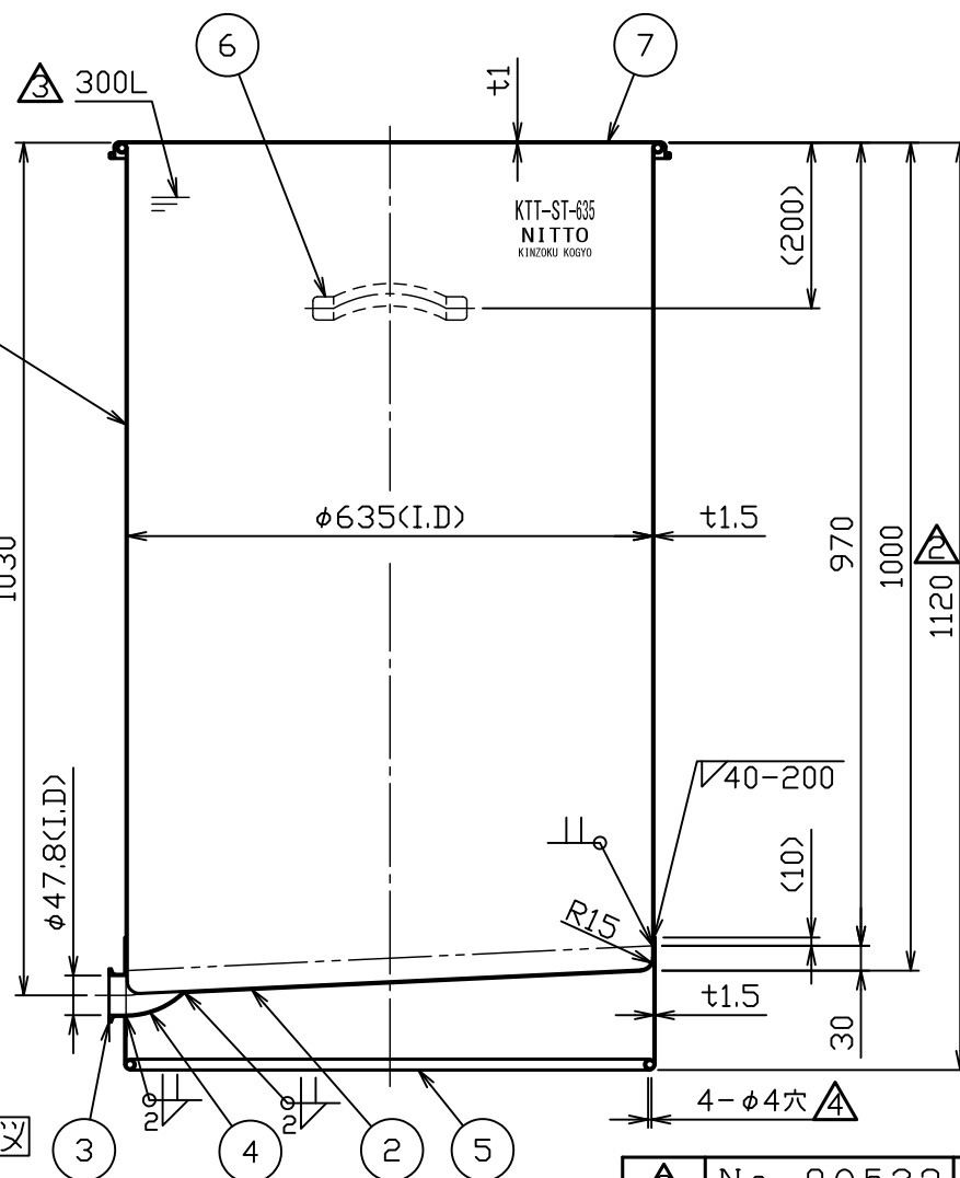
A-A断面図
