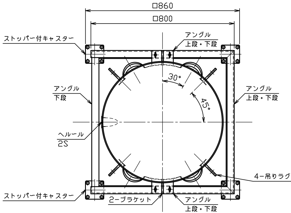
△蝶ボルト部詳細図 S = 1 : 4
