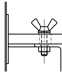
蝶ボルト部詳細図 S = 1 : 2
