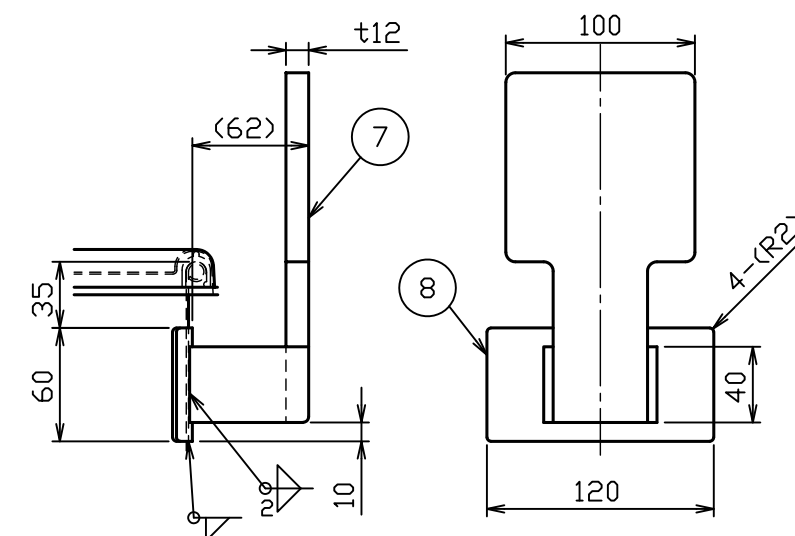
A 部詳細図 S = 1 : 4
