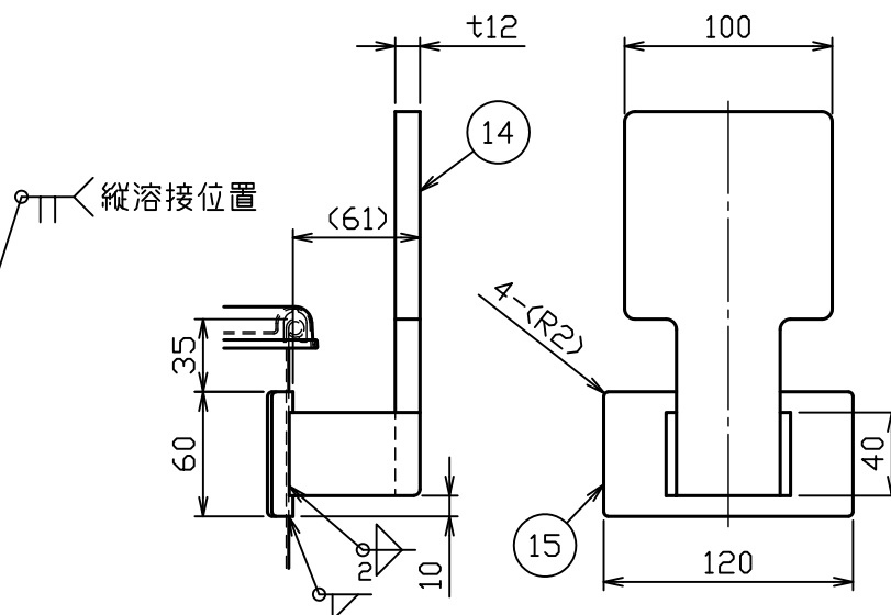
A部詳細図 S = 1 : 4
