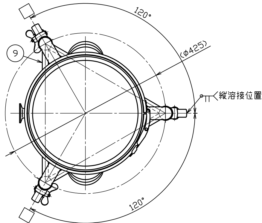
A部詳細図 S = 1 : 1
