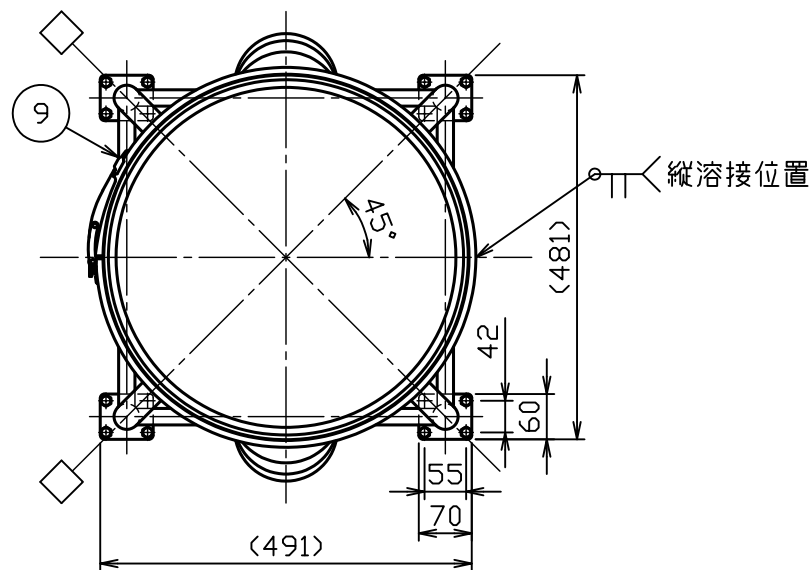
A部詳細図 S = 1 : 1
