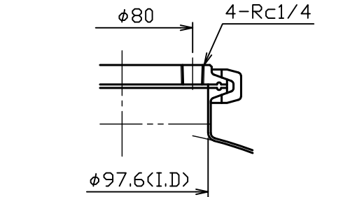
A部詳細図 S = 1 : 3
