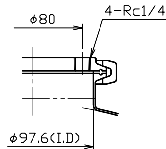
A部詳細図 S = 1 : 3
