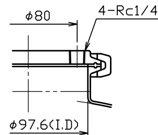
A部詳細図 S = 1 : 3
