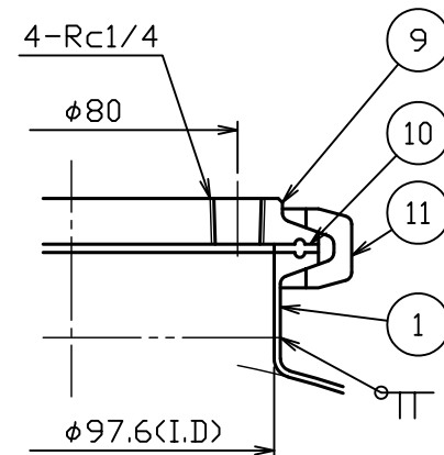
A部詳細図 S = 1 : 2
