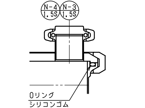
A部詳細図 S = 1 : 3
