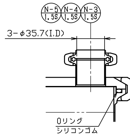
A部詳細図 S = 1 : 3
