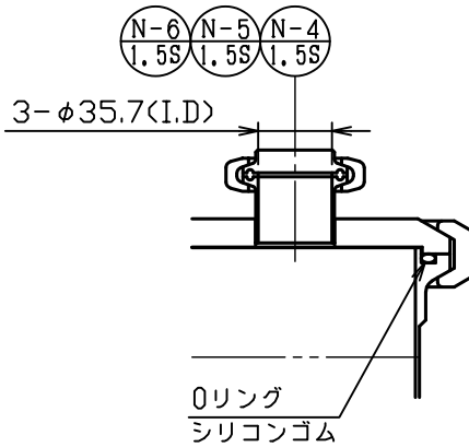
A部詳細図 S = 1 : 4
