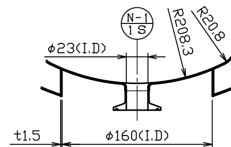
ドレン部詳細図 S = 1 : 4
