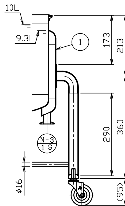
ドレン部詳細図 S = 1 : 4
