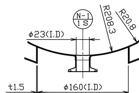
ドレン部詳細図 S = 1 : 4
