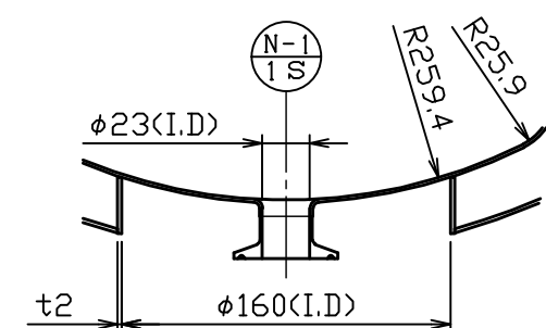
ドレン部詳細図 S = 1 : 4
