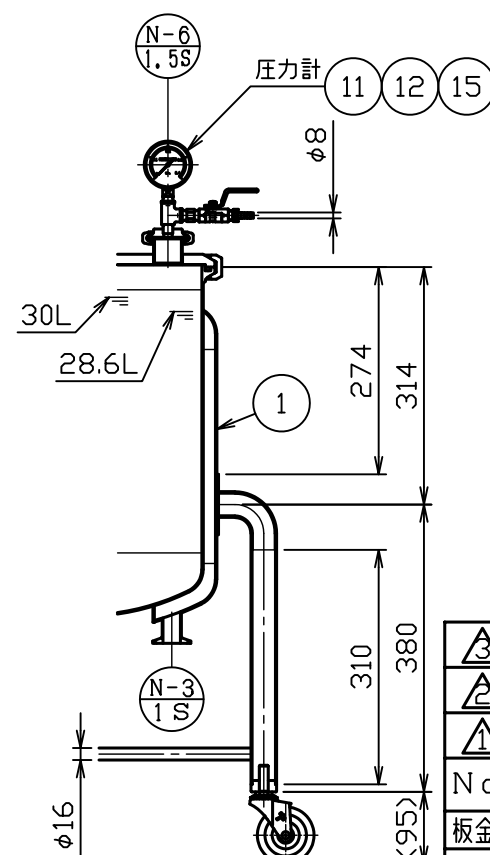
ドレン部詳細図 S = 1 : 4
