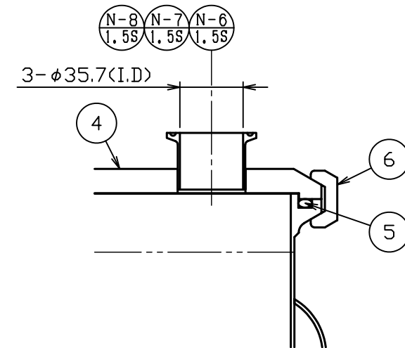
A部詳細図 S = 1 : 3
