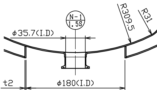
ドレン部詳細図 S = 1 : 4
