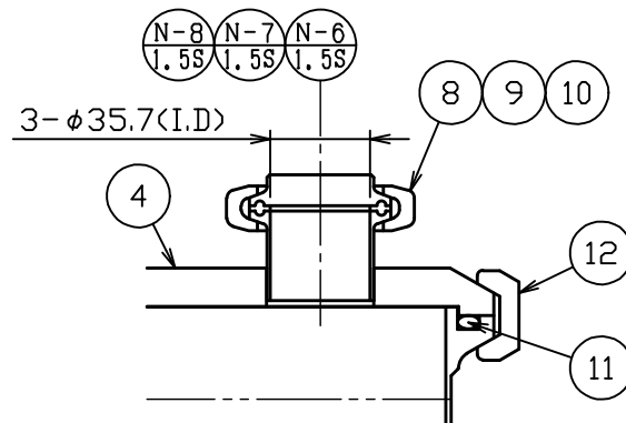
A部詳細図 S = 1 : 3
