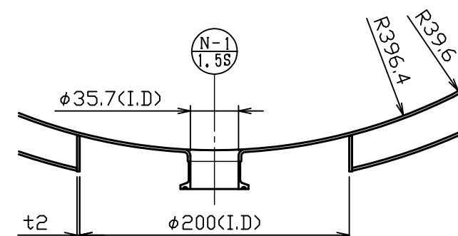
ドレン部詳細図 S = 1 : 4
