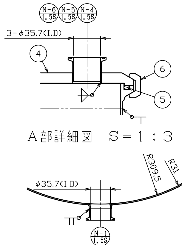
ドレン部詳細図 S = 1 : 4
