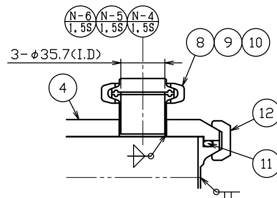
A部詳細図 S = 1 : 3
