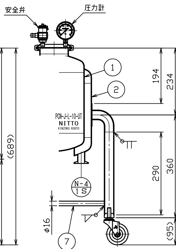
ドレン部詳細図 S = 1 : 4
