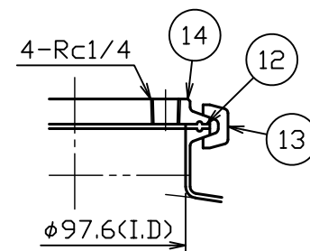
A部詳細図 S = 1 : 3
