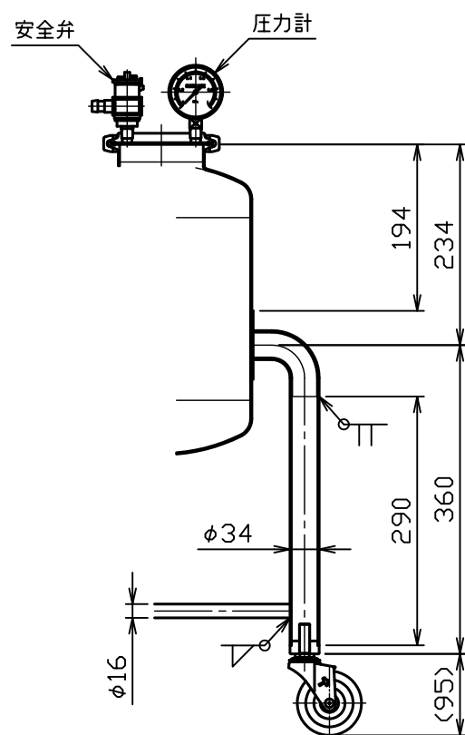
ドレン部詳細図 S = 1 : 4
