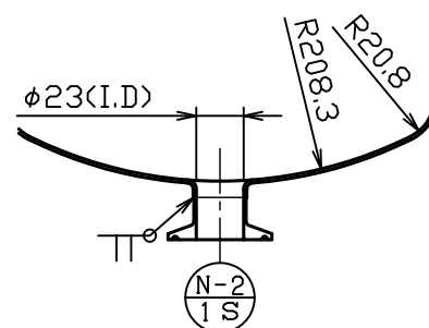
ドレン部詳細図 S = 1 : 4
