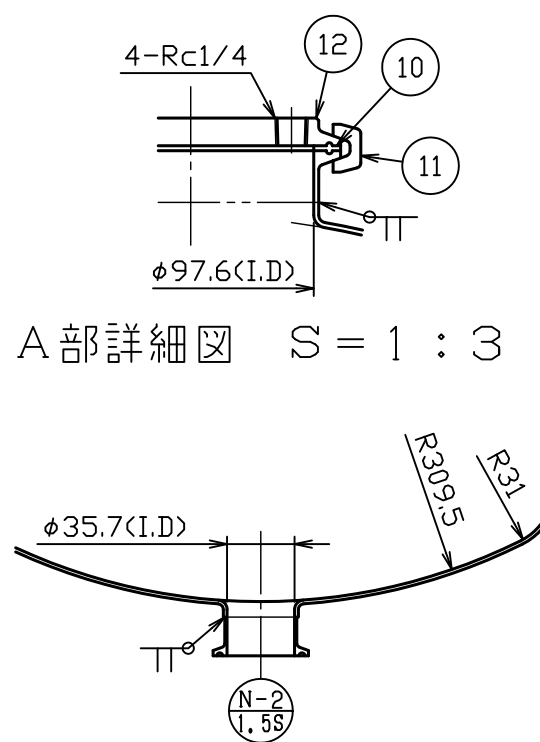
ドレン部詳細図 S = 1 : 4
