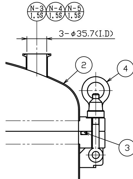
A部詳細図 S = 1 : 4
