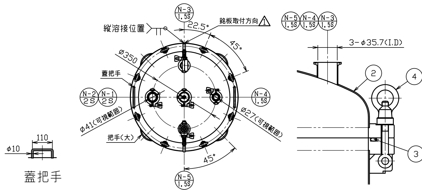
A部詳細図 S = 1 : 4
