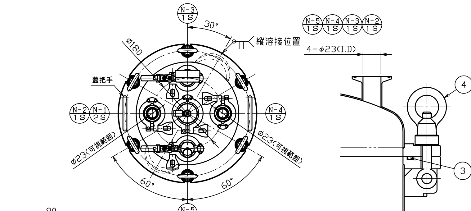
A部詳細図 S = 1 : 3
