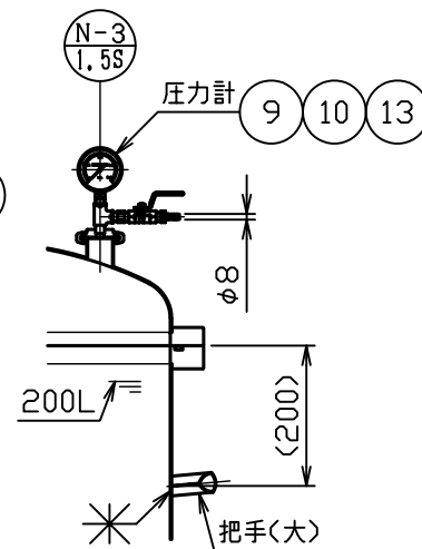
A部詳細図 S = 1 : 4
