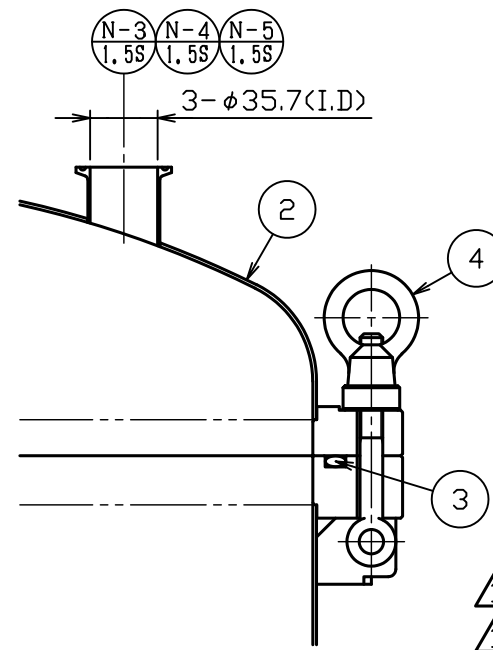
A部詳細図 S = 1 : 4
