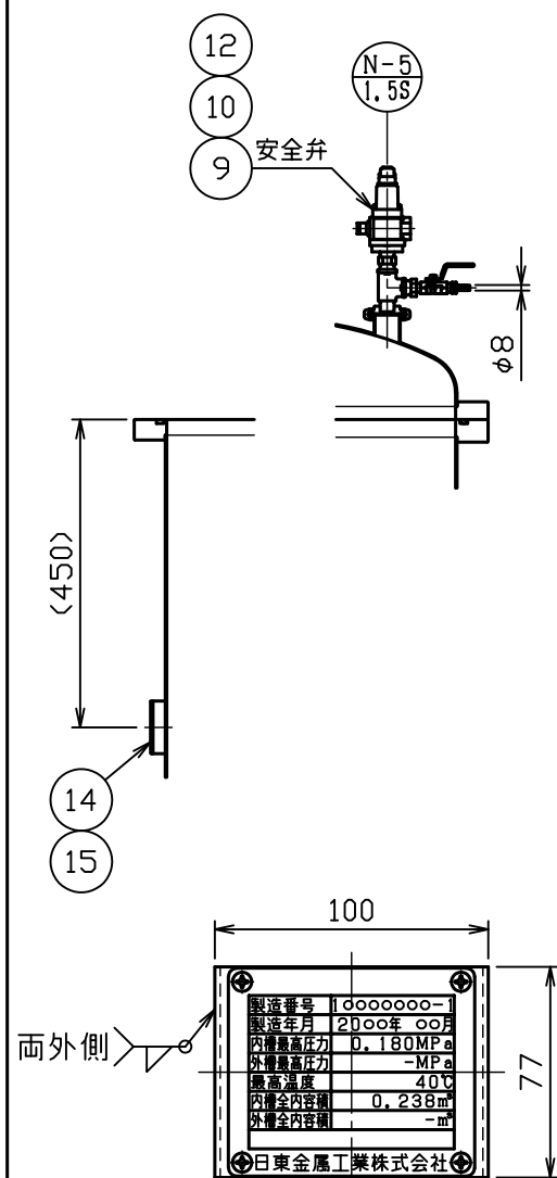
△ 銘板詳細図 S = 1 : 3
