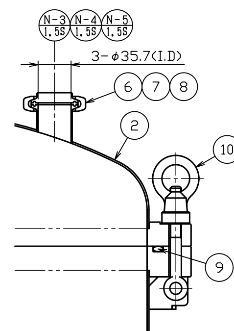
A部詳細図 S = 1 : 4
