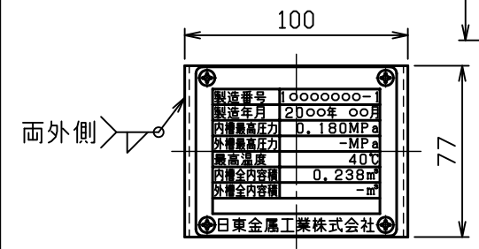
△ 銘板詳細図 S = 1 : 3
