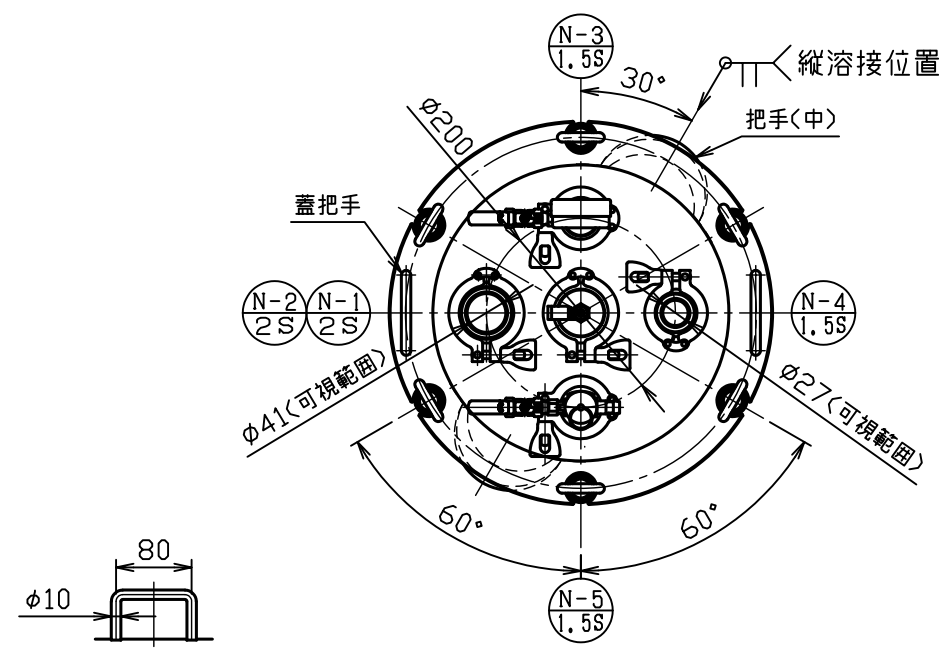
蓋把手
