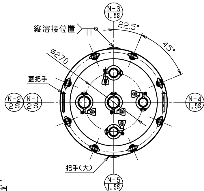
蓋把手
