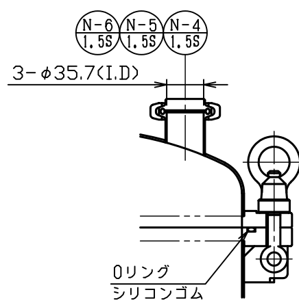
A部詳細図 S = 1 : 5
