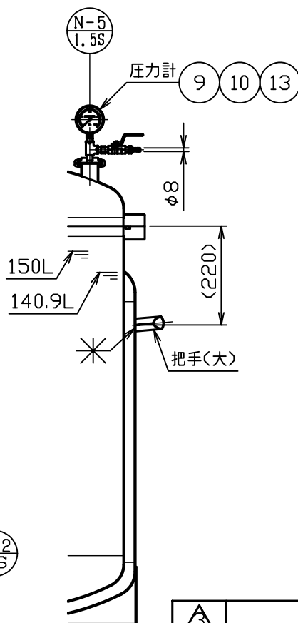
A部詳細図 S = 1 : 4
