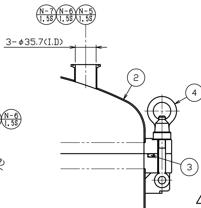
A部詳細図 S = 1 : 4
