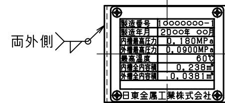
銘板詳細図 S = 1 : 3
